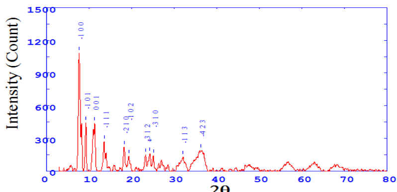
Fig: 3: FeZn (SB) 2 (H 2 O) 2 .
